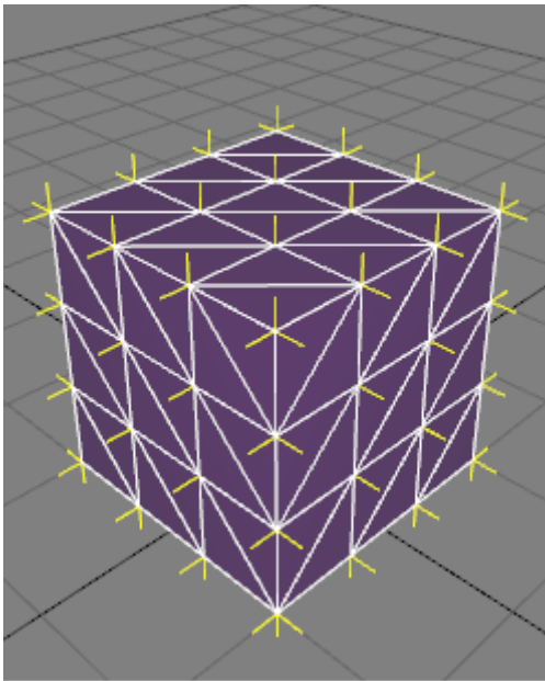
在盒上应用 85°的阈值角度的重新计算法线函数的结果。
