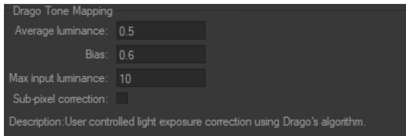
Drago 色调映射效果的选项。
