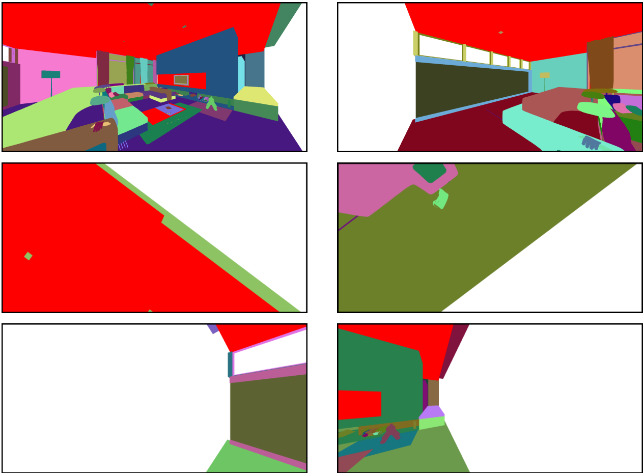
执行渲染以识别表面内部具有自动定向功能的每个表面的方向。上：向前和向后。中间：上下。底部：左侧和右侧。
