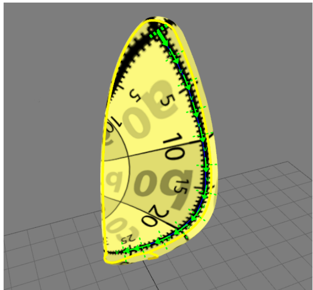
多-constraints method.
