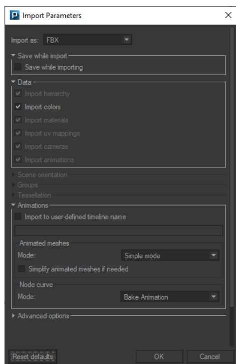
FBX 文件的“导入参数”对话框
