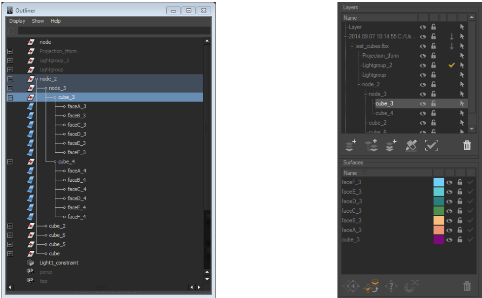
Maya (左) 和 Patchwork 3D (右) 中.fbx 格式的数据的图层层级结构。
