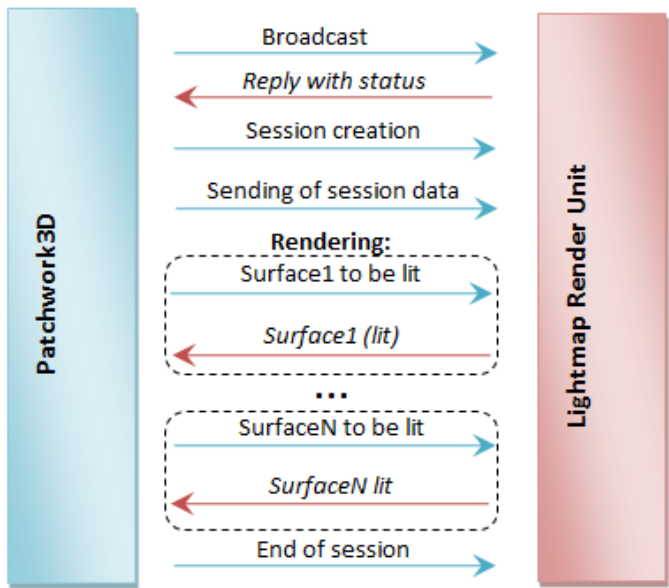
Patchwork 3D 和 Patchwork 光照渲染机之间的网络事件。
