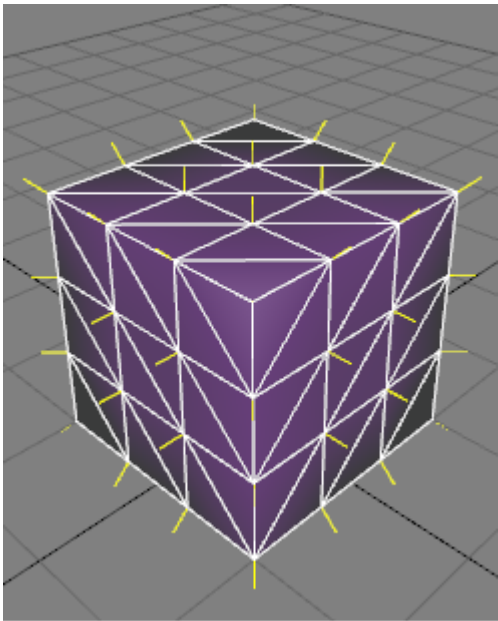
将盒子上的阈值角度为 95°的重新计算法线函数应用的结果。
