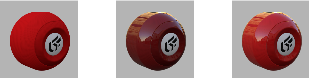
Filtrage de reflet sans texture de modulation. De gauche à droite : couche diffuse, couche de réflexion sans texture spéculaire, et résultat avec effet d'éclaircissement.
