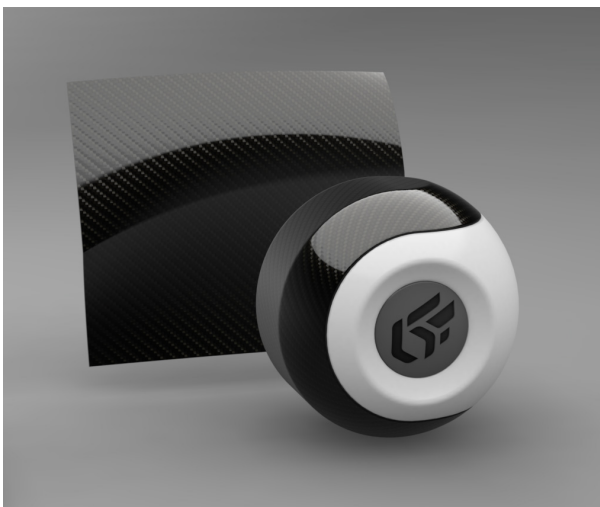
Rendu matériau.
