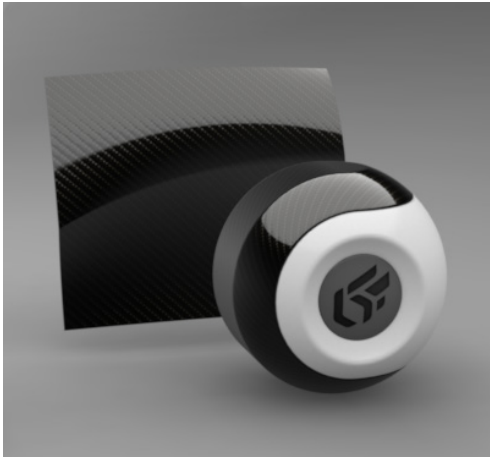
Image initiale.
