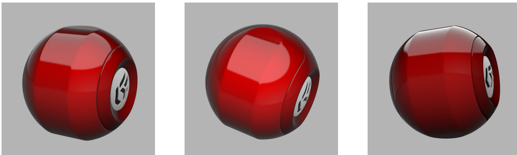
フレネル効果あり (屈折率 = 1.518)。
