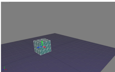
立方体のピボットの初期位置。
