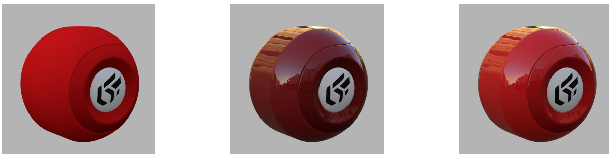
反射フィルタリング (変調画像なし)。左から右ディフューズレイヤー、反射レイヤー (変調画像なし)、ライトニング効果を使用した画像。
